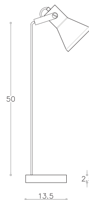
LUMINÁRIA DE MESA TAÇA
