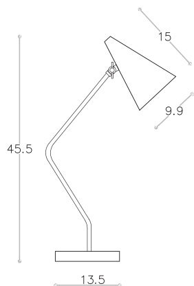
LUMINÁRIA DE MESA Ísis Soft
